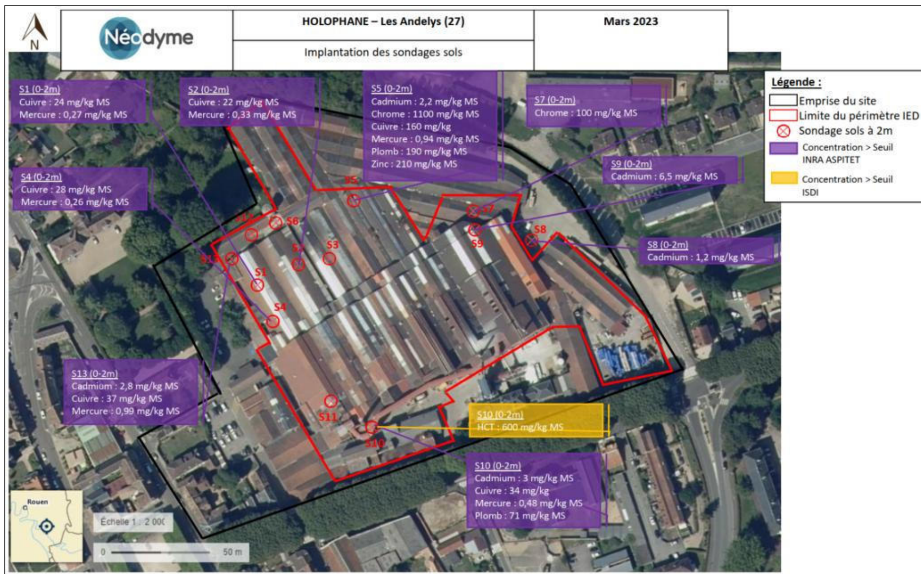
Figure 1 : Localisation des investigations et anomalies retenues dans les sols dans le périmètre IED du site (rapport NEODYME n°R-MAC-2303-1a du 28/03/2023)
