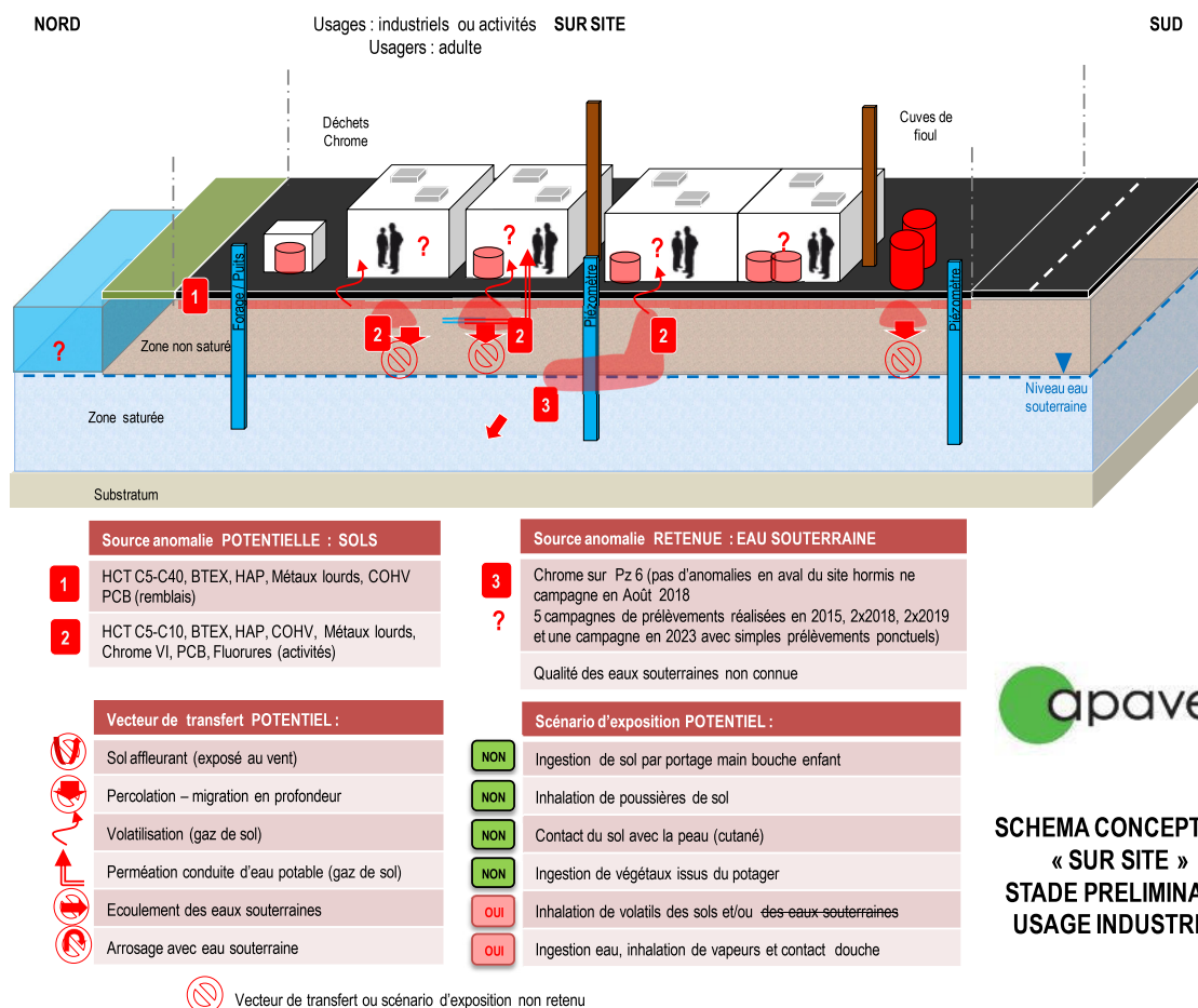
Figure 19 : Schéma conceptuel « SUR SITE » – stade préliminaire
