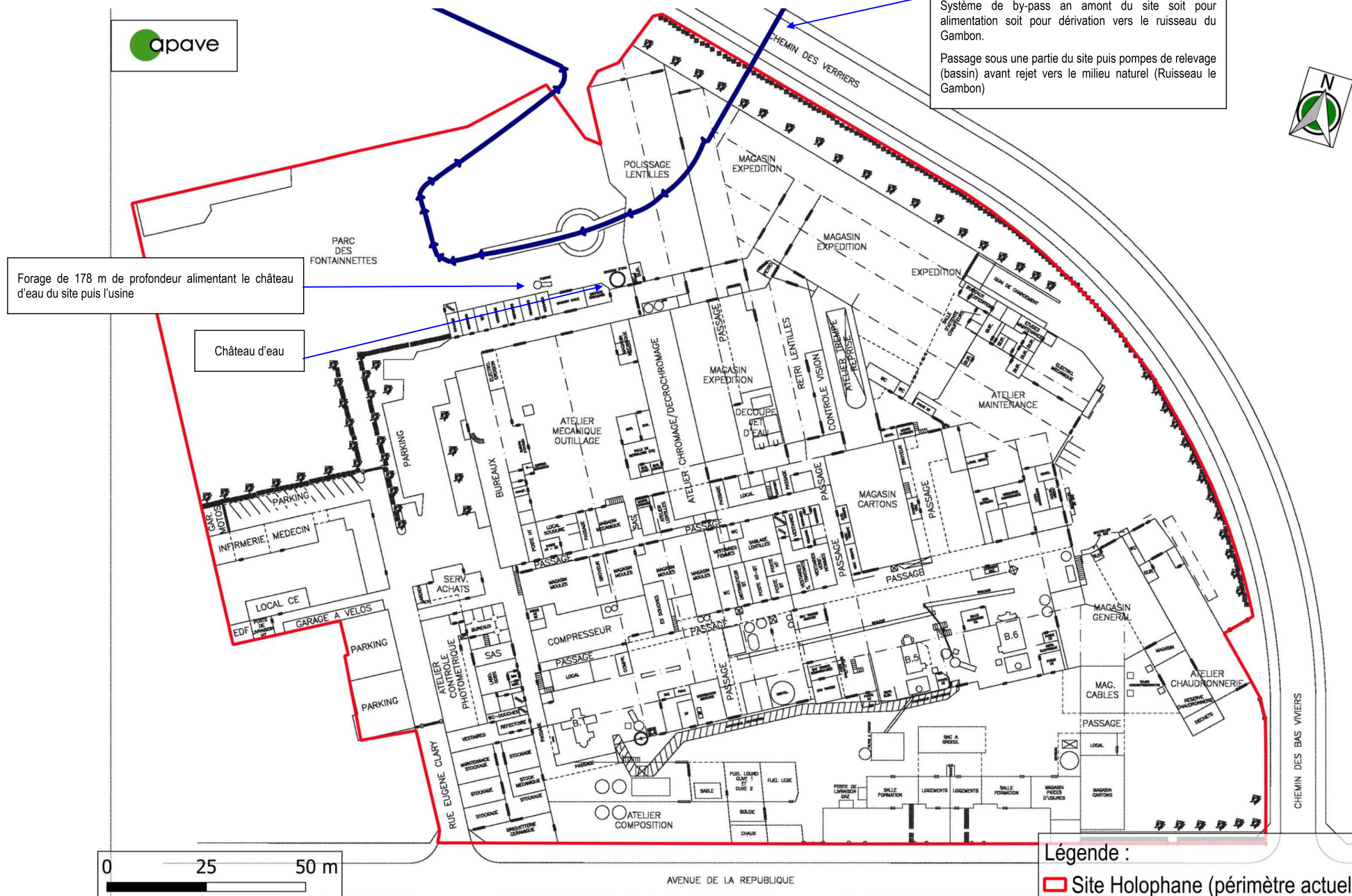
Figure 9 : Plan masse du site d'étude localisant les activités
