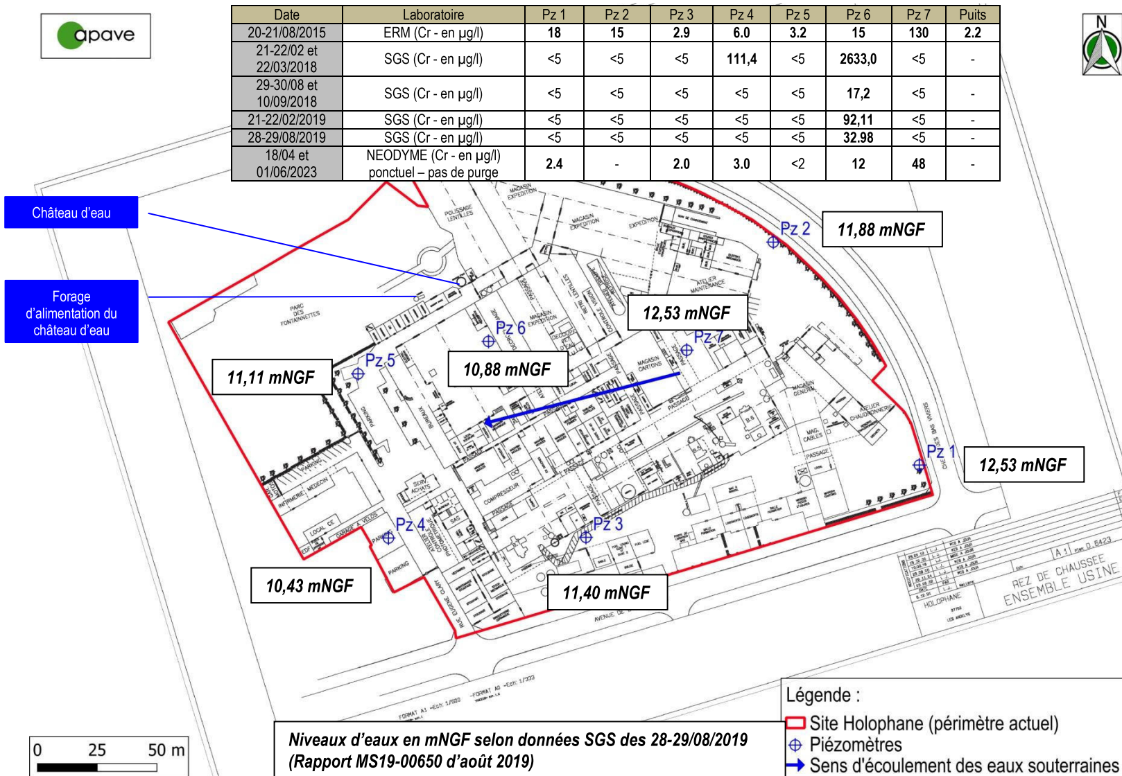
Figure 15 : Sens d'écoulement estimé de la nappe au droit du site selon données SGS (rapport MS19-00650 d'Août 2019)
